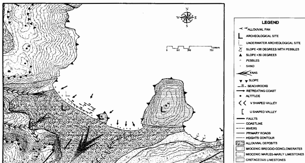
Σχήμα. 3 Γεωμορφολογικός χάρτης του Ίστρου
