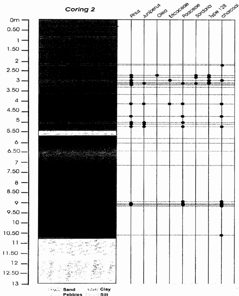
Σχήμα 7. Παλυνολογικό διάγραμμα της Γεώτρησης 2
