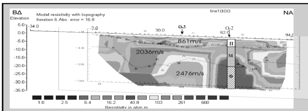
Σχήμα 6. Υπέρθεση του μοντέλου ταχύτητας της σεισμικής γραμμής Σ.Δ-1 πάνω στην γεωηλεκτρική τομή HT-1. Η γεώτρηση O-2 διάτρησε προσχώσεις (Π), μάργες (M) και την αποσαθρωμένη ζώνη της φυλλιτικής-χαλαζιτικής σειράς (Φ).
