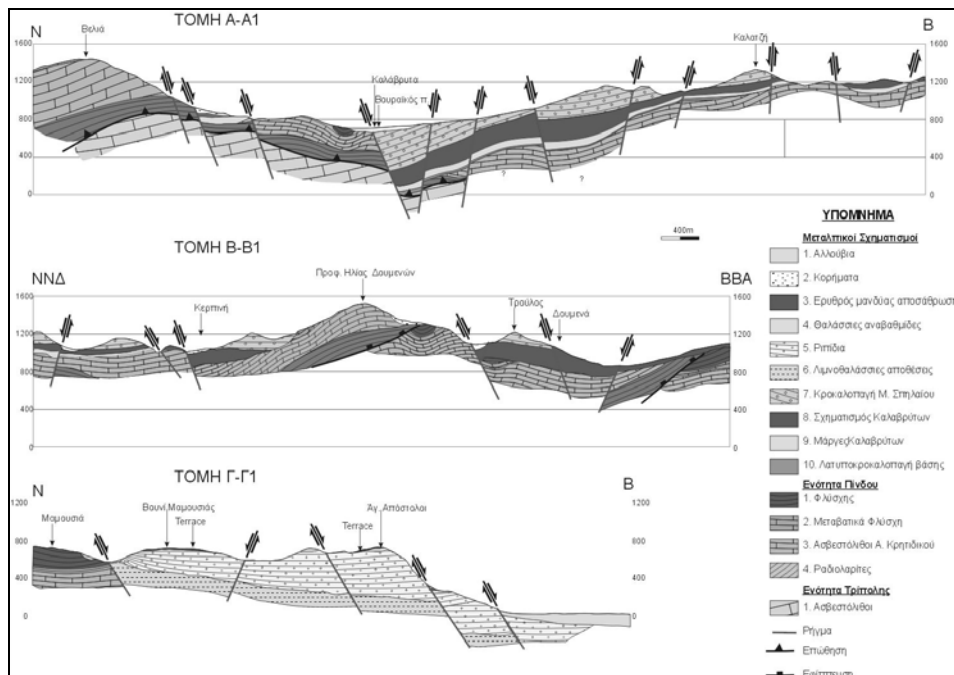
Εικ.3. Ενδεικτικές γεωλογικές τομές του φύλλου ΑΙΓΙΟ, από το νότιο τμήμα (Α-Α 1 ), κεντρικό (Β-Β 1 ), και βόρειο (Γ-Γ 1 ). Στις τομές εμφανίζονται επιμέρους στρώματα των αλπικών και μεταλπικών σχηματισμών, που διακρίθηκαν από τη γεωλογική χαρτογράφηση.
