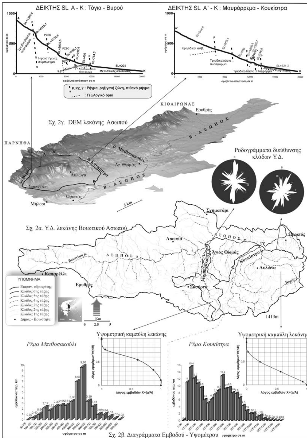
Σχήμα 2. Μορφοτεκτονική ανάλυση ανατολικής λεκάνης Βοιωτικού Ασωπού.
