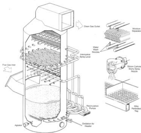
Σχήμα 1. Σχηματική απόδοση διάταξης που περιλαμβάνει τα βασικά εξαρτήματα από τα οποία απαρτίζεται ένας πύργος αποθείωσης καπναερίων. Πηγή: (Nolan, 2000).
