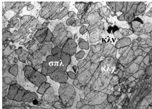
Σχήμα 5. Skarn, αποτελούμενο από κρυστάλλους κλινοχουμίτη (κλχ) και κρυστάλλους σπινελίου (σπλ) μέσα σε κλινόχλωρο (κλν). Διερχ. φως, // πρίσματα, x10.
