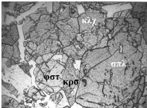
Σχήμα 10. Ιδιόμορφος κρύσταλλος παρασιτικής κεροσίλβης (κρσ) σε επαφή με σπινέλιο (σπλ), με φοροστερίτη (φστ) και με κλινοχουμίτη (κλχ). Διερχ. φως, // πρίσματα, x20.
