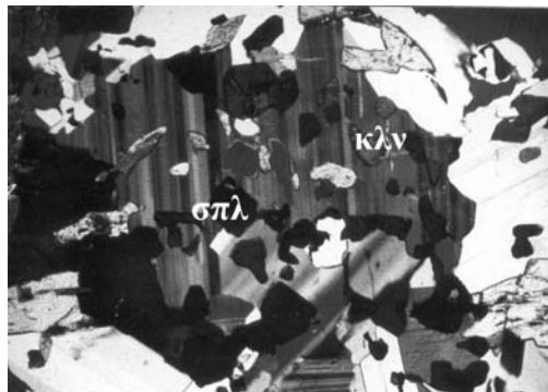
Σχήμα 13. Μεγάλος κρύσταλλος κλινόχλωρου με χαρακτηριστικές λαμέλλες, περικλείοντας κρυστάλλους σπινελίου (σπλ). Διερχ. φως, κάθετα πρίσματα, x20.
