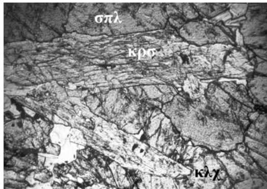
Σχήμα 11. Δύο ιδιόμορφοι κρύσταλλοι παρασιτικής κεροσίλβης (κρσ) μέσα σε μάζα από κλινοχουμίτες και σπινέλιους. Διερχ. φως, // πρίσματα, x20.
