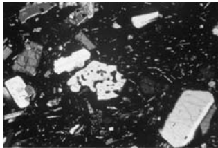
Σχήμα 5. Μικροφωτογραφία τραχυτικής λάβας δείχνει δύο τύπους πλαγιοκλάστων: μαγματικά διαβρωμένα (στο κέντρο) και υγιή (κάτω δεξιά), βιοτίτη και πυρόξενο εντός μικροκρυσταλλικής κύριας μάζας (#11s, μήκος φωτογραφίας 2.2 mm)
