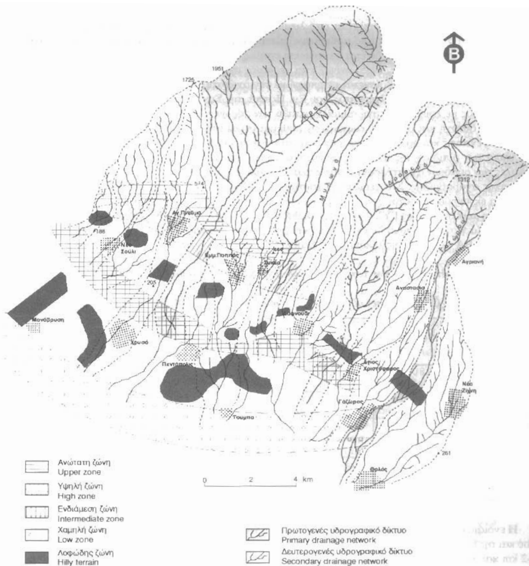
Εικόνα 1. Υδρογραφικό δίκτυο, λεκάνες απορροής των χειμάρρων και ζώνες απόθεσης σύνθετων αλλουβιακών ριπιδίων στην περιοχή ΝΑ Μενικίου – ΒΑ λεκάνης Σερρών.
