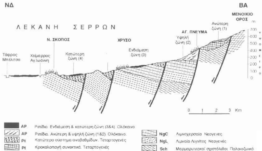
Εικόνα 3. Σχηματική γεωλογική τομή του ΝΑ Μενοικίου - λεκάνης Σερρών. Figure 3. Schematic geological profile of the SW Menikio - NE Serres basin.
