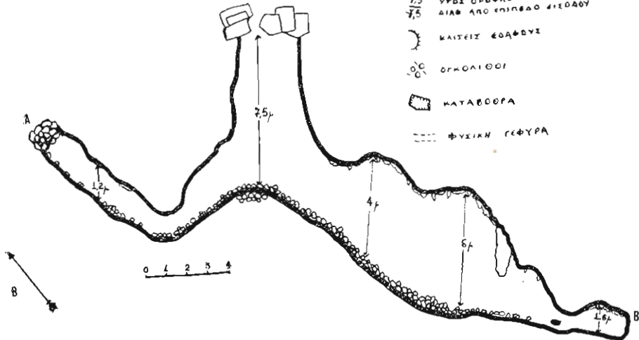
Ἄνω Κάτωψις καὶ κάτω Τομή τοῦ Σπηλαιο - βάραθρου «Προφήτης Ἡλίας» Ἄνω Γλυφάδας Ἀριθ. 2.
