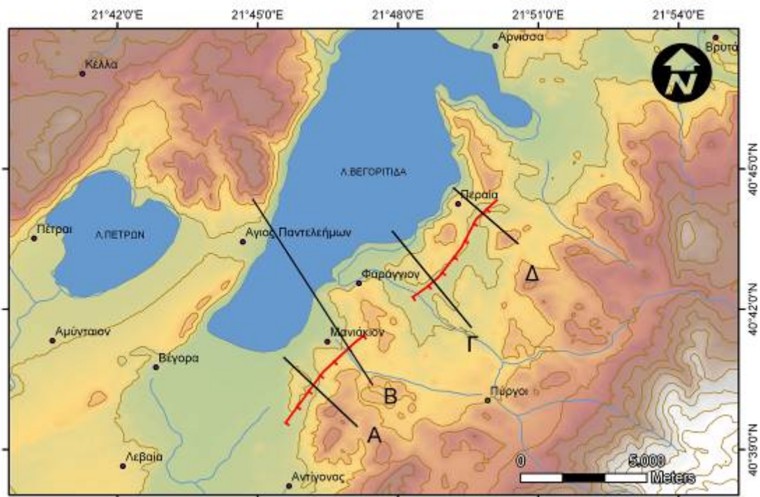
Σχ.4.3.4.4 Ψηφιακό μοντέλο αναγλύφου, διακρίνεται το ρήγμα Περαιάς-Μανιάκι. Ισοϋψείς ανά 100m (επάνω) και οι μορφολογικές τομές που έχουν εξαχθεί από αυτό (κάτω).
