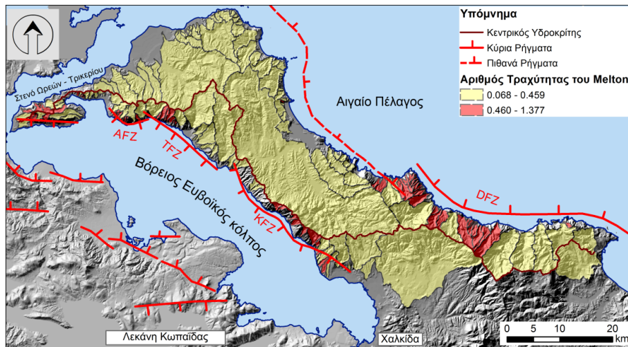
Εικόνα 8. Χωρική κατανομή των τιμών του αριθμού τραχύτητας του Melton στη βόρεια Εύβοια (DFZ: Ρηξιγενής ζώνη Διρφύος, KFZ: Ρηξιγενής ζώνη Κανδηλίου, TFZ: Ρηξιγενής ζώνη Τελέθριου, AFZ: Ρηξιγενής ζώνη Αιδηψού).
