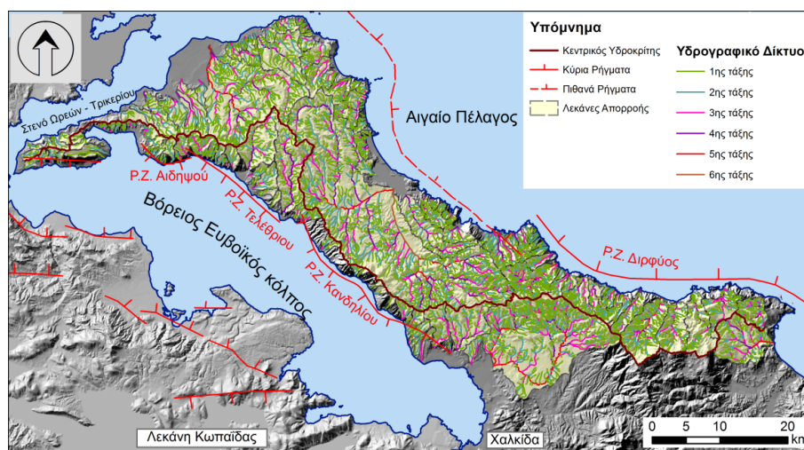
Εικόνα 3. Χάρτης των υδρογραφικών δικτύων και των αντίστοιχων λεκανών απορροής της περιοχής μελέτης. Στην χάρτη φαίνονται επίσης οι κύριες ρηξιγενείς ζώνες καθώς και ο κεντρικός υδροκρίτης της βόρειας Εύβοιας.
