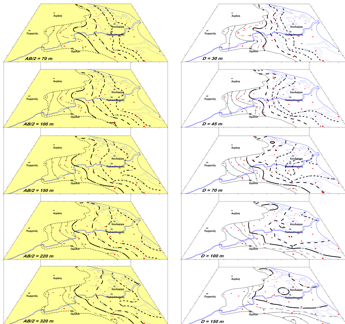
Εικόνα 3. Χάρτες οριζόντιας κατανομής της φαινόμενης ειδικής ηλεκτρικής αντίστασης για AB/2 = 70 , 100, 150, 220 και 320 μέτρα (αριστερά) και οι αντίστοιχοι χάρτες οριζόντιας κατανομής της ηλεκτρικής ειδικής αντίστασης για τα βάθη των 30, 45, 70, 100 και 150 μέτρων (δεξιά).
