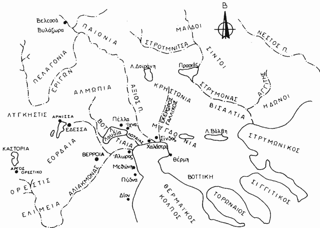
Σχ.1. Η Μακεδονία και ο Θερμαϊκός στην εποχή του Σπαρτιά (1ος αιώνας π.Χ.). Χημική Βιβλιοθήκη Θεσσαλονίκης - Τμήμα Γεωλογίας, Α.Π.Θ.
