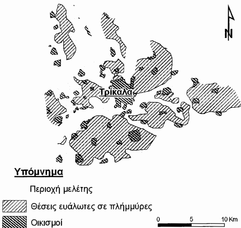
Σχήμα 5: Χάρτης πλημμυρικής επικινδυνότητας σε σχέση με τις πόλεις και τους οικισμούς στην περιοχή μελέτης (πεδιάδα Τρικάλων - Κалаμπάκας).
