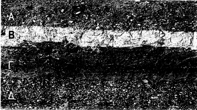
Φωτ. 1: Εδαφικός ορίζοντας από εκσκαφή στη πόλη των Τρικάλων, στον οποίο φαίνονται επιχώσεις (Α) στον ανώτερο ορίζοντα, δύο στρώσεις λεπτής γης (Β & Γ) και μια ανάμικτη στρώση χαλικών και λεπτής γης (Δ).
