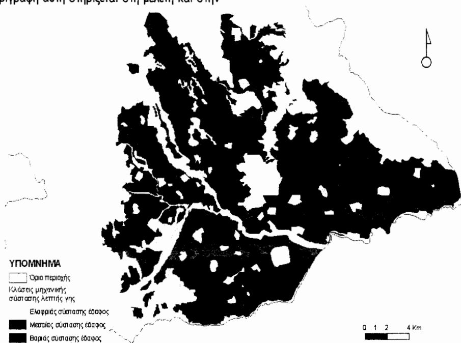
Σχήμα 3: Συνθετικός χάρτης κατάταξης των εδαφών στη πεδιάδα Τρικάλων - Καλαμπάκας, βασισμένος σε στοιχεία του Ι.Χ.Τ.Ε.Α. και τους χάρτες Κλάσεων Εδαφών, κλίμακας 1:50.000, φύλλα «Τρίκαλα», «Καλαμπάκα», «Μουζάκι» και «Καρδίτσα», έκδοσης 1999 του Ι.Χ.Τ.Ε.Α., καθώς και σε παρατηρήσεις κατά την εργασία υπαίθρου (Μπαθρέλλος 2005).
