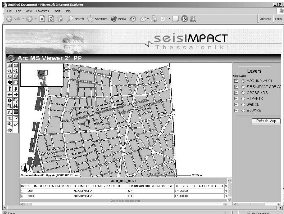
Σχήμα 4. Ενδεικτική μακέτα (mockup) οθόνης του συστήματος
