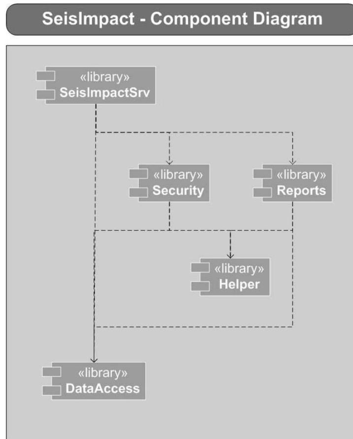
Σχήμα 3. Διάγραμμα στοιχείων (Component Diagram)
