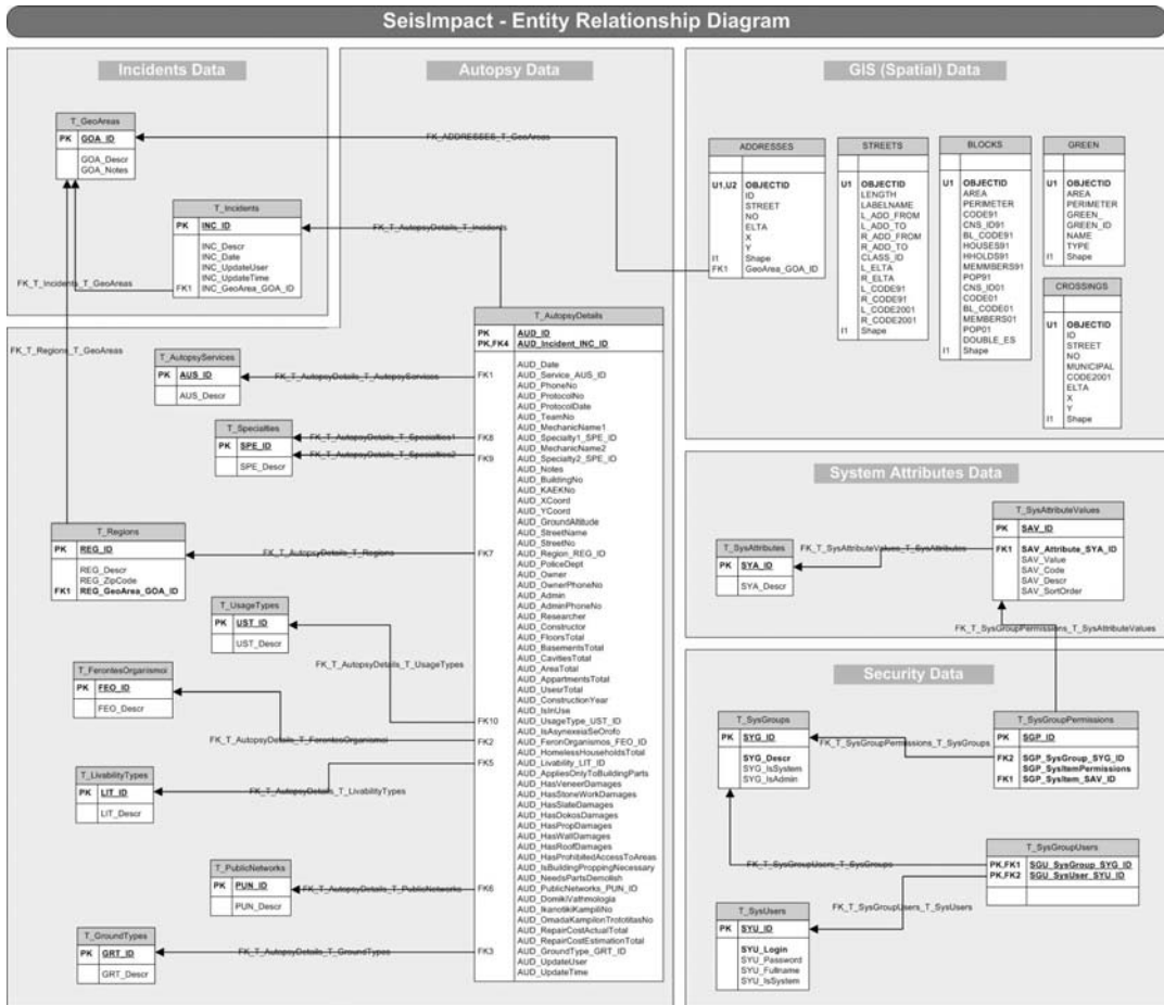
Σχήμα 2. Διάγραμμα συσχέτισης (Entity Relationship Diagram)
