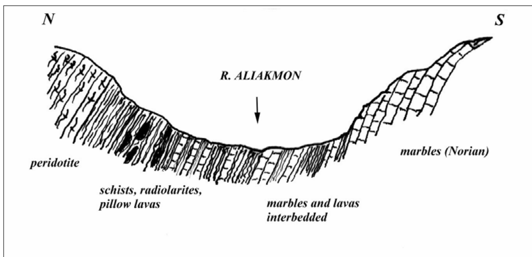
Σχήμα 3. Γεωλογική τομή δυτικά και ανάντι της Μονής Ζαμπόρντα. Geological section to the west and upside of Zabordas monastery.
