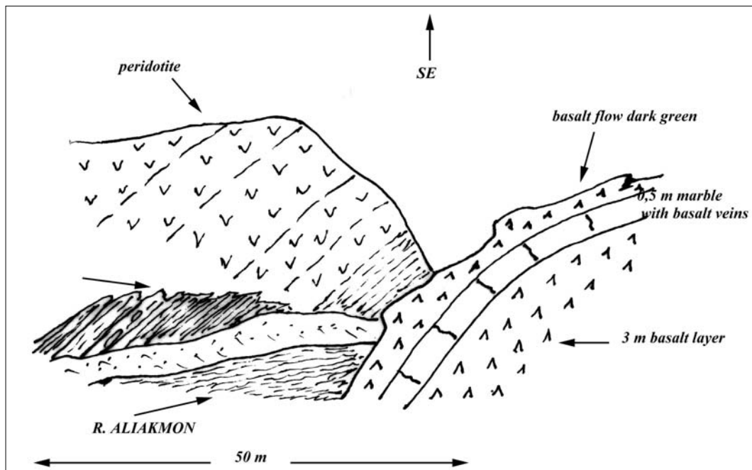
Σχήμα 1. Σκαρίφημα των σχηματισμών, δεξιά όχθη του Αλιάκμονος, 2 χλμ ανάντι της Μονής Ζαμπόρντα σε ευθεία γραμμή. Schedule of geological section, right shore of Aliakmon valley, 2 km upslope of Zabordas monastery.
