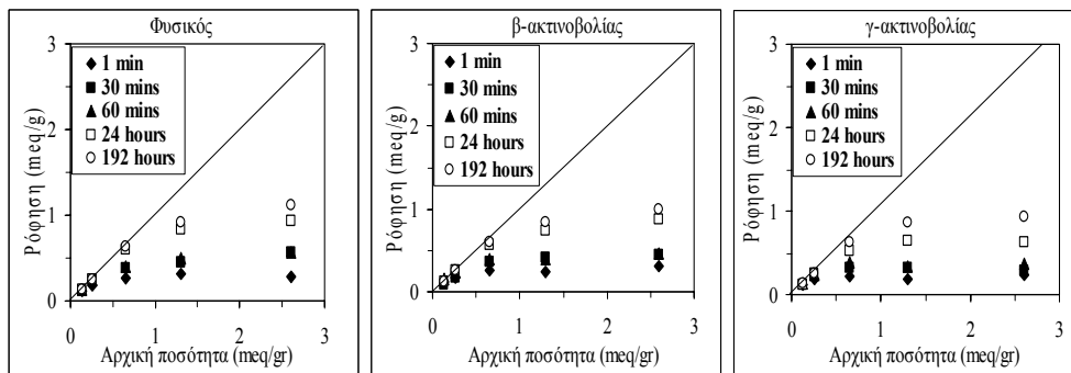
Σχήμα 5. Διαγράμματα ρόφησης Sr^{2+} σε σχέση με το χρόνο για φυσικό κλινοπυλίθιθος, για κλινοπυλίθιθος επεξεργασμένο με ακτινοβολία ηλεκτρονίων και κλινοπυλίθιθος επεξεργασμένο με ακτινοβολία-γ. (άξονας x: αρχική ποσότητα γραμμοισοδύναμων στο διάλυμα, άξονας y: γραμμοισοδύναμα τα οποία ροφήθηκαν, για όλες τις συγκεντρώσεις έγινε αναγωγή ανά γραμμάριο κλινοπυλίθιθου)
