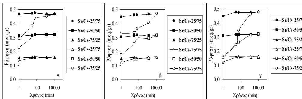
Σχήμα 7. Ρόφηση Cs + (μαύρα σύμβολα) και Sr 2+ (κενά σύμβολα) α) σε φυσικό κλινοπυλίλιθο β) σε κλινοπυλίλιθο επεξεργασμένο με ακτινοβολία ηλεκτρονίων (10 14 e/cm 2 ) γ) σε κλινοπυλίλιθο επεξεργασμένο με ακτινοβολία-γ (70Mrad). Τα ίδια σχήματα αναφέρονται σε διαλύματα αντίστοιχων αναλογιών για παράδειγμα ο μαύρος κύκλος αναφέρεται σε διάλυμα αναλογίας Cs + / Sr 2+ =75/25 και ο κενός κύκλος σε διαλύματα Sr 2+ /Cs + =75/25. Συγκέντρωση διαλύματος 0,5xCEC.
