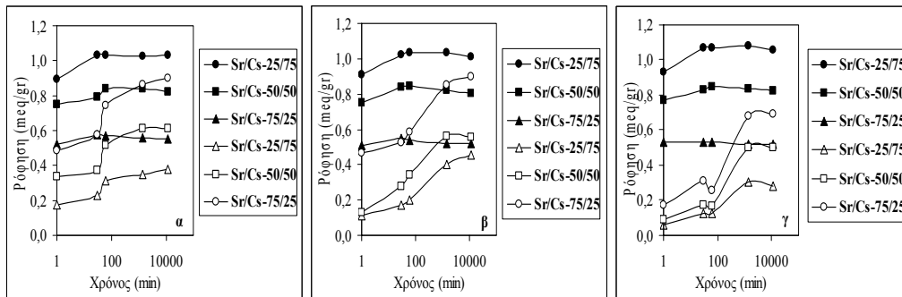
Σχήμα 6. Ρόφηση Cs + (μαύρα σύμβολα) και Sr 2+ (κενά σύμβολα) α) σε φυσικό κλινοπυλίλιθο β) σε κλινοπυλίλιθο επεξεργασμένο με ακτινοβολία ηλεκτρονίων (10 14 e/cm 2 ) γ) σε κλινοπυλίλιθο επεξεργασμένο με ακτινοβολία-γ (70Mrad). Τα ίδια σχήματα αναφέρονται σε διαλύματα αντίστοιχων αναλογιών για παράδειγμα ο μαύρος κύκλος αναφέρεται σε διάλυμα αναλογίας Cs + / Sr 2+ =75/25 και ο κενός κύκλος σε διαλύματα Sr 2+ /Cs + =75/25. Συγκέντρωση διαλύματος 2xCEC.
