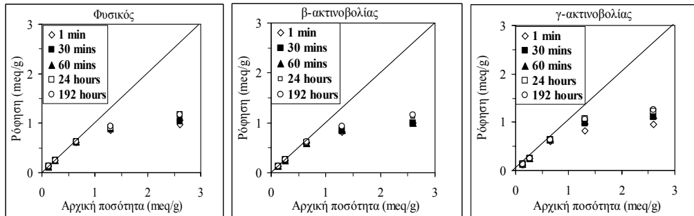
Σχήμα 4. Διάγραμμα ρόφησης Cs^+ σε σχέση με το χρόνο για φυσικό κλινοπυλίθιθος, για τροποποιημένο κλινοπυλίθιθος με ακτινοβολία ηλεκτρονίων και κλινοπυλίθιθος τροποποιημένο με ακτινοβολία-γ. (άξονας x: αρχική ποσότητα γραμμοισοδύναμων στο διάλυμα, άξονας y: γραμμοισοδύναμα τα οποία ροφήθηκαν, για όλες τις συγκεντρώσεις έγινε αναγωγή ανά γραμμάριο κλινοπυλίθιθου)
