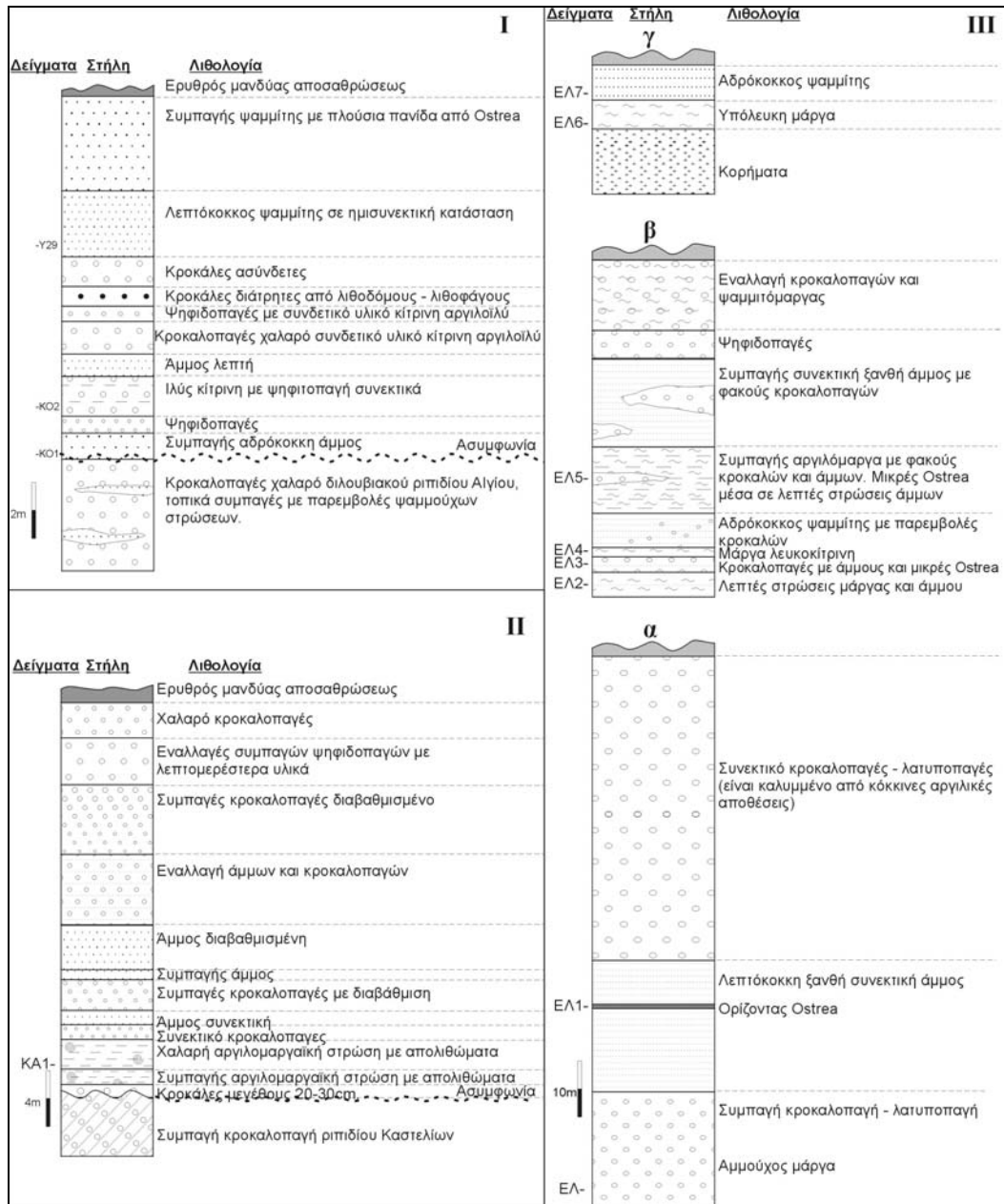
Εικ. 2. Στρωματογραφικές στήλες θαλάσσιων αναβαθμιδών περιοχής Λάκας Κουνινών (I), Καστελιών (II) και Ελίκης (III).
