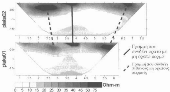
Σχ.3 Εικόνες αντιστροφής των τομογραφικών οδεύσεων plaka01 και plaka02. Με συνεχή γραμμή συνδέεται ορατός κορμός (τομογραφία plaka01) με πιθανή συνέχειά του και με διακεκομμένη γραμμή συνδέονται πιθανοί μη ορατοί στόχοι που διακρίνονται στις δύο παράλληλες τομογραφίες.
