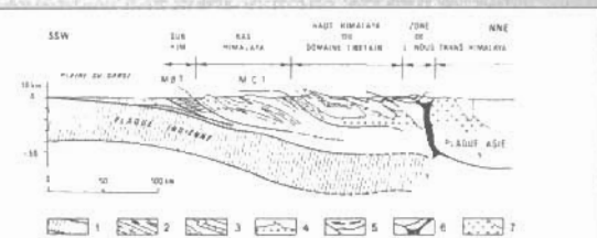
Εικ. 2. Σχηματική τομή των Ιμαλαίων.
