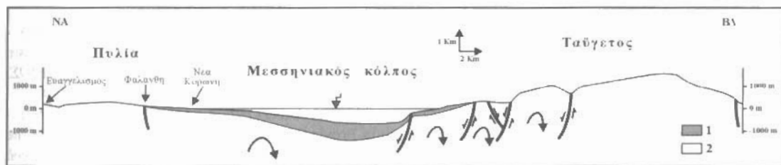
1:Μεταλλικά ιζήματα, 2:Προνεογενές υπόβαθρο. Fig. 4.: Schematic cross-section A-A'-A'' across Messinias gulf and Taygetos mountain. 1:Post-alpine sediments, 2:Pre-neogene basement.
