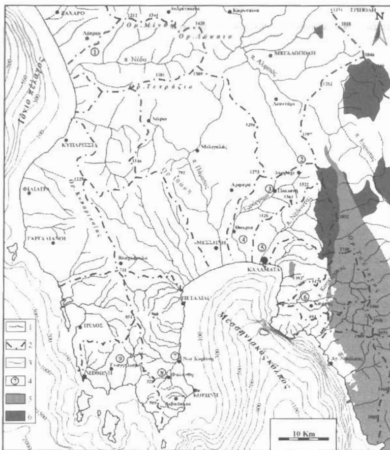
Εικ. 2. Οι θέσεις εμφάνισης των μεταλικών σχηματισμών, που περιέχουν κροκάλες από μεταμορφωμένα πετρώματα, στη ΝΑ Πελοπόννησο. 1:υδρογραφικό δίκτυο, 2:υδροκρίτες, 3:ισοβαθείς, 4:θέσεις εμφάνισης, 5:ενότητα Μάνης, 6:ενότητα Άρνας.
