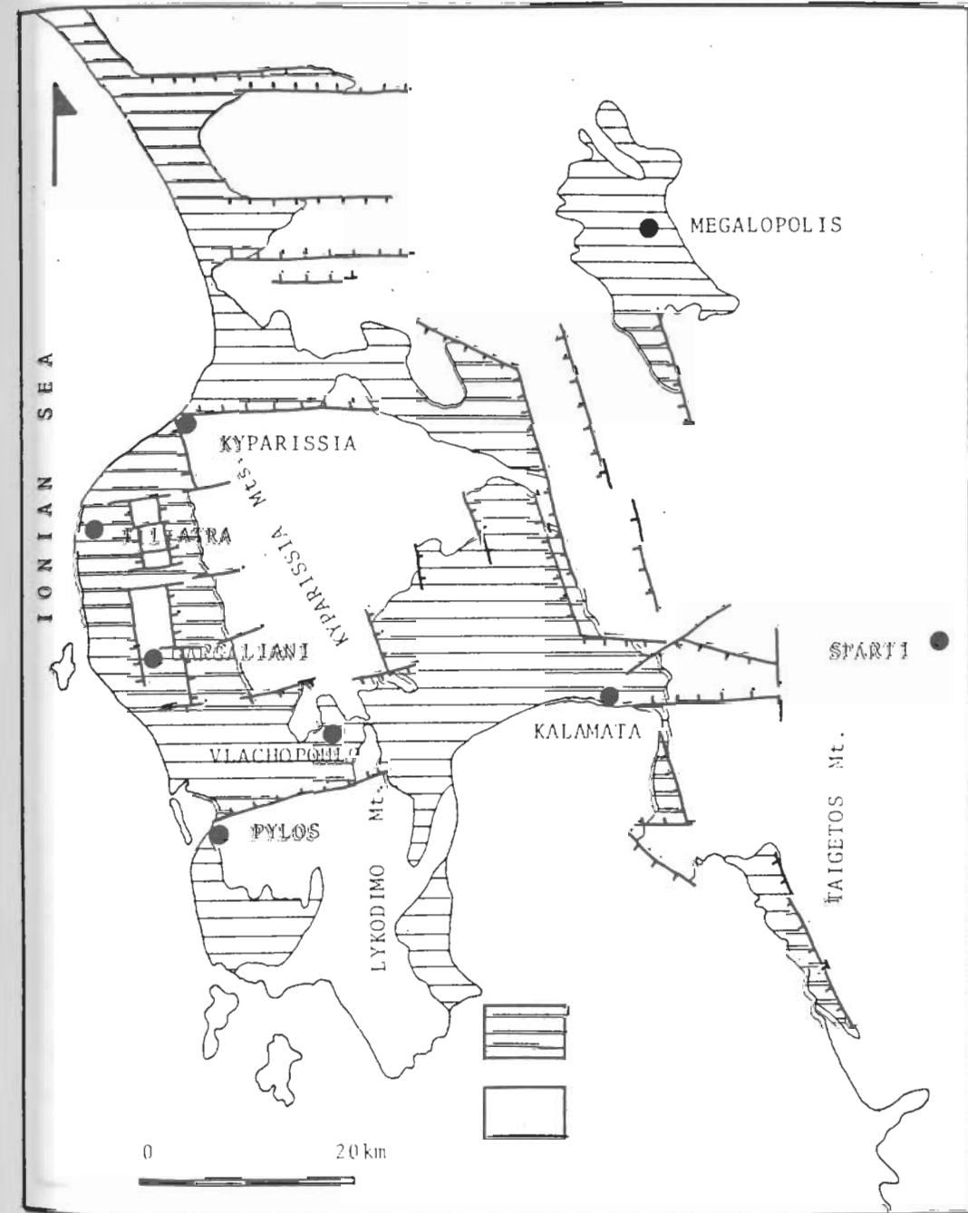
Εικ. 4. Οι 1ης τάξης νεοτεκτονικές μακροδομές. Fig. 4. Neotectonic macrostructures of 1st order.
