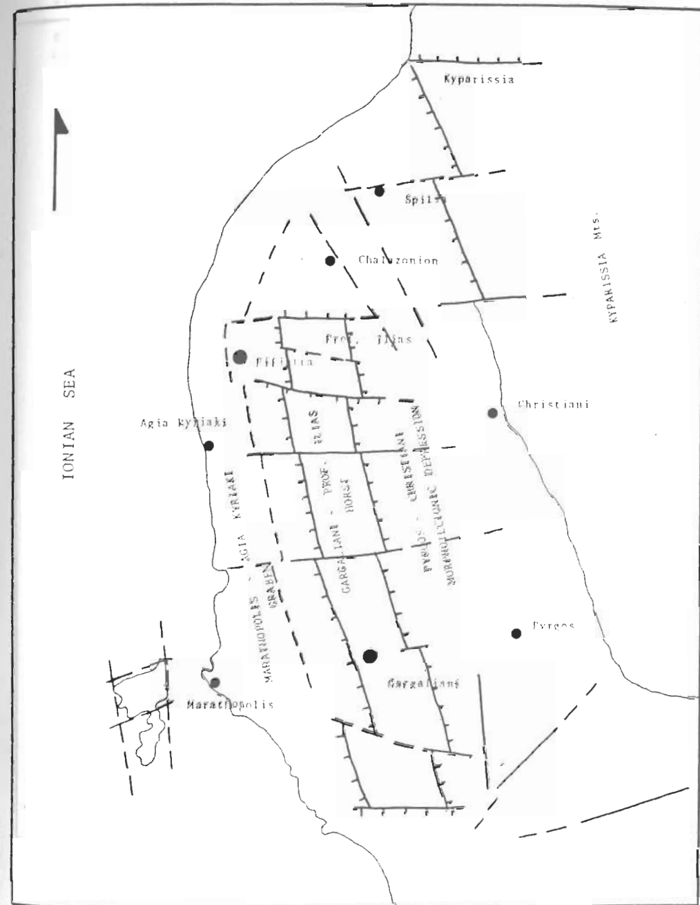
Εικ. 5. Οι ΙΙης τάξης νεοτεκτονικές μακροδομές. Fig. 5. Neotectonic macrostructures IIInd order.
