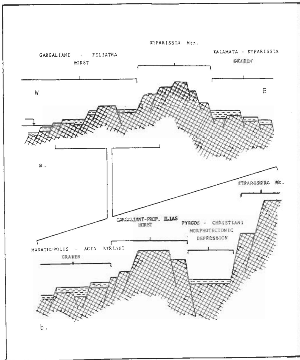
Εικ. 6. Σχηματικές τομές α. Των Ιης τάξης νεοτεκτονικών μακροδομών β. Των ΙΙης τάξης νεοτεκτονικών μακροδομών
