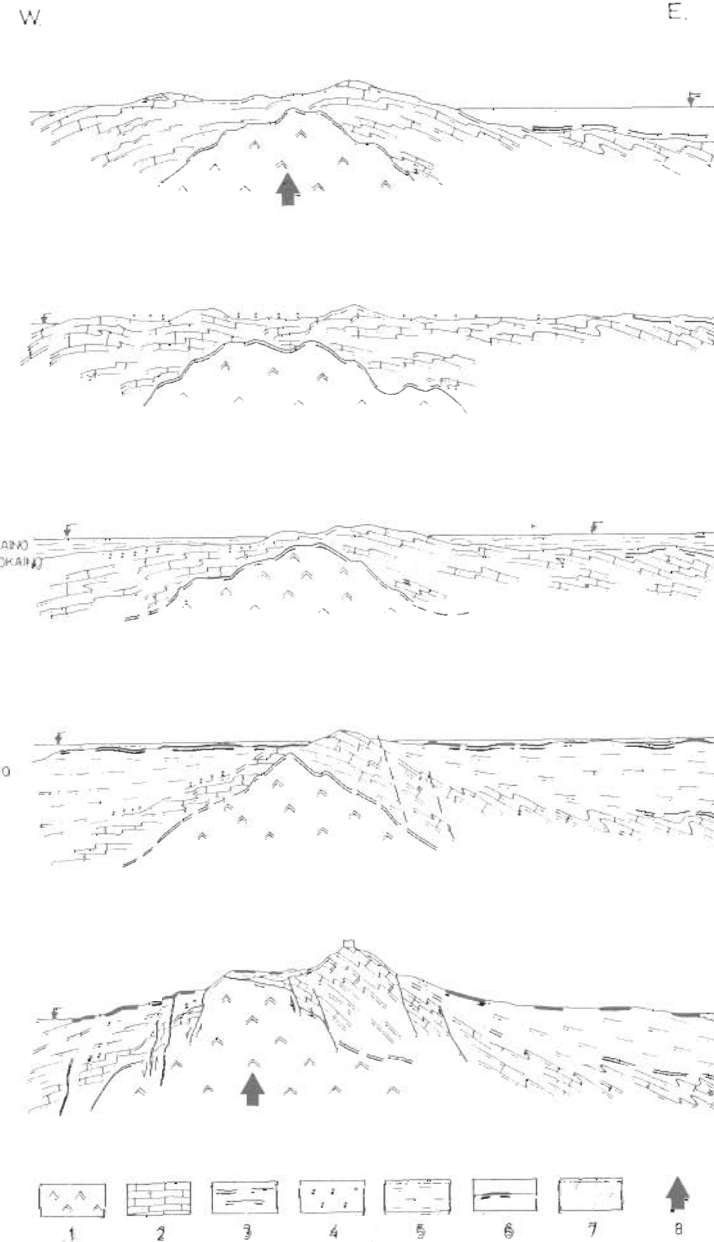
Εικ. 8. Σχηματική απεικόνιση της νεοτεκτονικής δομής και εξέλιξης της χερσονήσου της Κυλλήνης: 1: Εβαπορίτες, 2: Σχηματισμός Ασβεστολίθων Κάστρου, 3: Σχηματισμοί Μέσου-Ανώτερου Μειόκαινου, 4: Κροκαλοπαγή Ψηλής Ράχης, 5: Σχηματισμός Ασβεστοψαμμιτών Γλώσσας, 6: Αλλούβια, 7: Ανοδικές κινήσεις - Διαπειρισμός.
