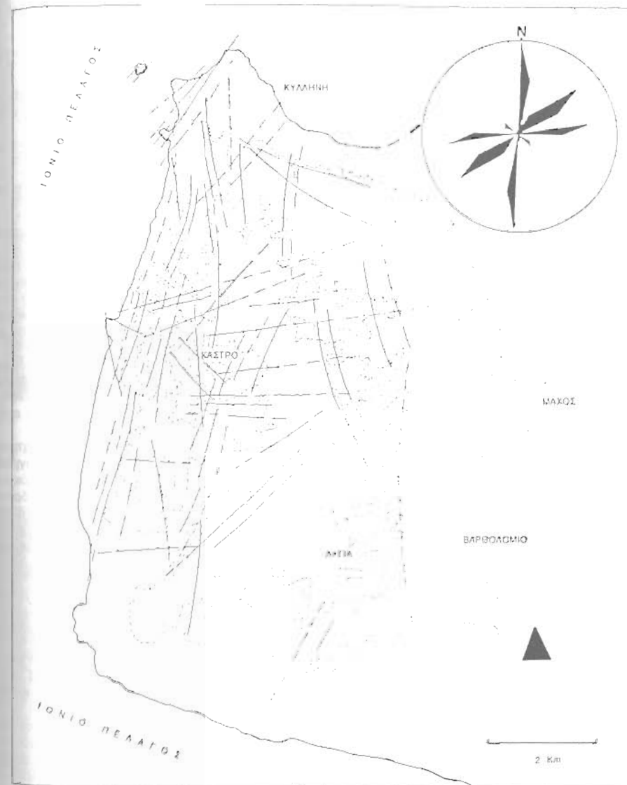
Εικ. 5. Ο ρηξιγενής ιστός της χερσονήσου της Κυλλήνης και τα 3 συστήματα διεύθυνσεων των ρηγμάτων.
