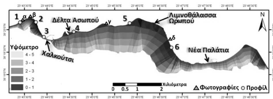
Σχήμα 2. Μορφολογία περιοχής και θέσεις τοπογραφικών τομών (1-6) & φωτογραφιών (α-δ).
