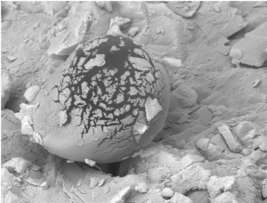
Σχήμα 11 - Μία περίεργη δομή, το «αυγό του Tissint», ανακλύφθηκε από τον καθηγητή Wallis από το Πανεπιστήμιο του Κάρντιφ στην Αγγλία. Τα σπασίματα στην επιφάνεια της σφαιρικής αυτής δομής αποτελούν σύμφωνα με τον συγγραφέα μία κοιλότητα που περιείχε άνθρακα και οξυγόνο, συστατικά απαραίτητα για την ανάπτυξη ζωής. Η μέγιστη διάμετρος του «αυγού» φθάνει τα 10 \mu\text{m} .
