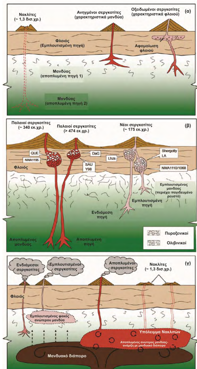
Σχήμα 2 - (α-γ) Μοντέλα προσωμοίωσης μαγματισμού στον πλανήτη Άρη. (α) Μοντέλο αφομοίωσης φλοιού (από Herd et al. , 2002). (β, γ) Μοντέλα πολλαπλών μανδυσικών πηγών (β: Symes et al. , 2008, γ: Blinova & Herd, 2009).
