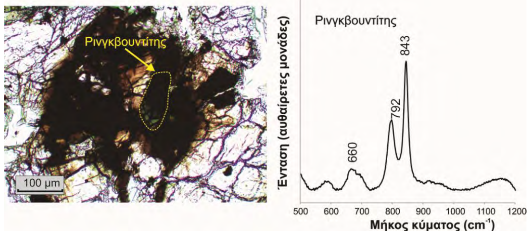
Σχήμα 9 – Αριστερά απεικονίζεται μία εικόνα που έχει ληφθεί από πετρογραφικό μικροσκόπιο. Φαίνεται ένα τμήμα του εσωτερικού του μετεωρίτη Tissint το οποίο έχει υποστεί πολύ υψηλές πιέσεις και θερμοκρασίες έπειτα από την πρόσκρουση αστεροειδούς στην επιφάνεια του πλανήτη Άρη. Το πράσινο ορυκτό, με το κίτρινο περίγραμμα, είναι το ορυκτό ρινγκβουντίτης. Αποτελεί το μεγαλύτερο σε μέγεθος ρινγκβουντίτη που έχει βρεθεί ποτέ σε μετεωρίτη. Η εφαρμογή της μικρο-φασματοσκοπίας Raman απέδειξε τη φύση αυτού του ορυκτού όπως απεικονίζεται στο χαρακτηριστικό φάσμα της δεξιάς εικόνας.
