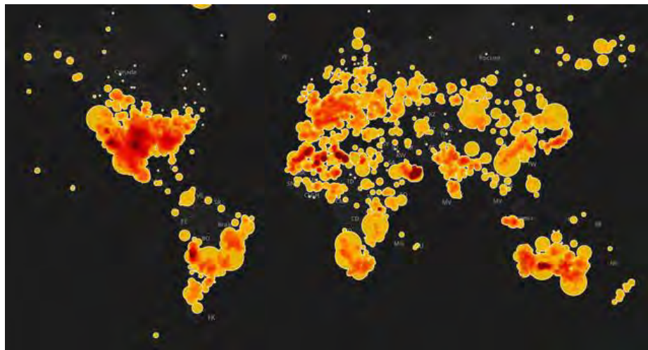
Σχήμα 6 – Θέσεις πτώσης μετεωριτών στη Γη τα τελευταία 4300 χρόνια. Στο χάρτη απεικονίζονται 34513 σημεία πρόσκρουσης.
