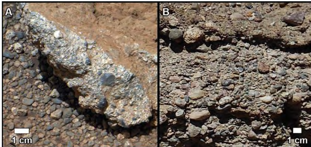
Σχήμα 10 – Σύγκριση κροκαλοπαγών από δύο διαφορετικούς πλανήτες. Α) Φωτογραφία που λήφθηκε από την κάμερα 100-mm Mastcam του οχήματος Curiosity στον πλανήτη Άρη. (Β) Γήινοι αποστρογγυλεμένοι κλάστες από αλλουβιακές αποθέσεις, όντας παρόμοιου μεγέθους και σχήματος με εκείνους της φωτογραφίας από τον πλανήτη Άρη (Ερημος Ατακάμα, Χιλή).
