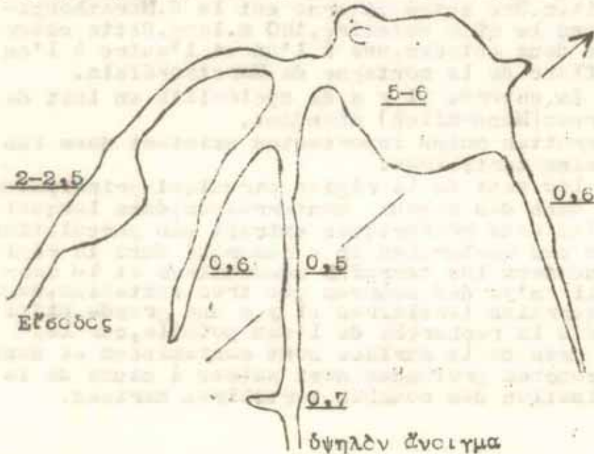
Κάτοψη της σπηλιάς "Κ Ε Ρ Α Τ Ο" Κλίμαξ 1:200
