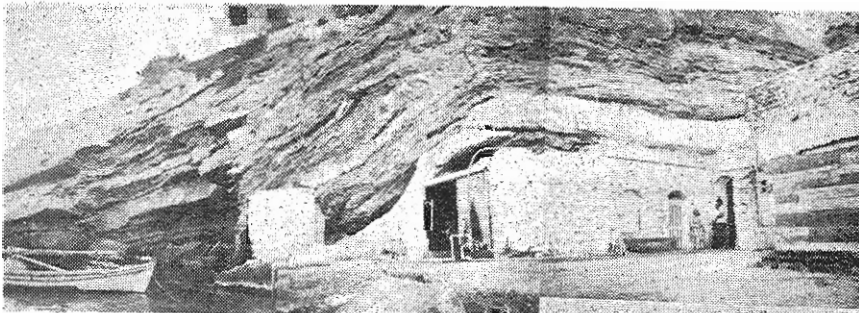
2- Σπήλαιον «Θερμὴ Πηγή» ἢ «Σπηλιὰ» Θερωῶν Ἰκαρίας. Φαίνεται καθαρὰ ἡ πτύχωσις τοῦ ἀσβεστολίθου καὶ τοῦ μαρμάρου κατὰ στρώσεις. Φωτ. Ἄνας Πετροχείλου
