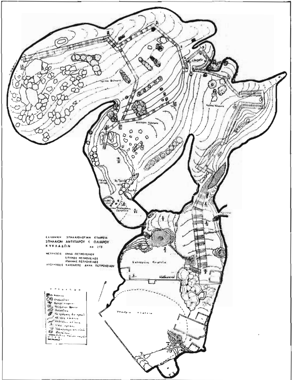
Εικ. 3. Κάτοψη του σπηλαιού 'Αντιπαρού ἢ 'Ωλιαροῦ, με τὴ χάραξη τῆς τουριστικῆς διαδρομῆς.
