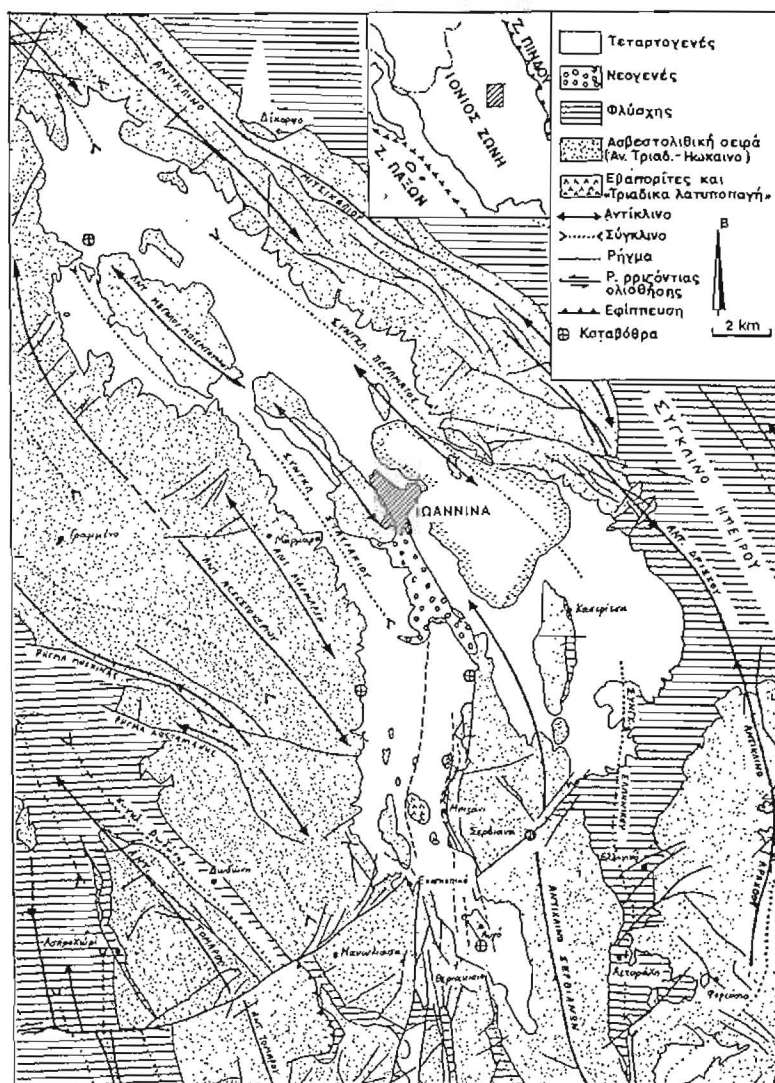
Σχ. 2: Τεκτονικός χάρτης της ευρύτερης περιοχής λεκανοπεδίου Ιωαννίνων (Καρακίτσιος 1994)
